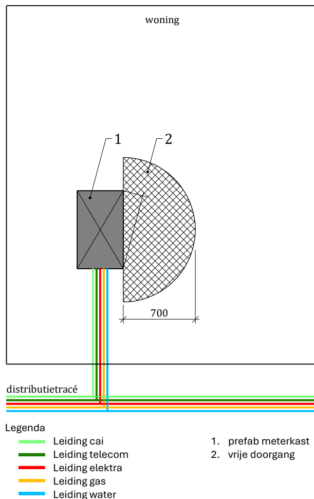
Figuur 1 - Werkruimte aan voorzijde prefab meterkast (bovenaanzicht)
